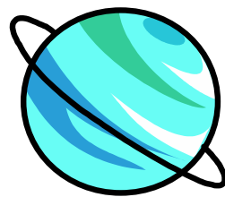
Planet
