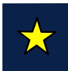
Stjärna
