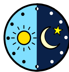
Dygn
