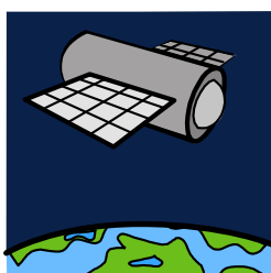
Satellit
