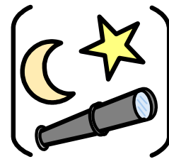
Astronomi
