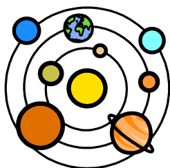
Solsystem
