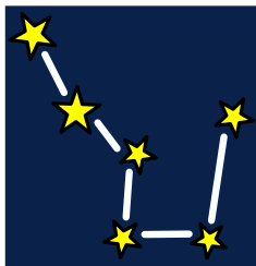
Stjärnbild
