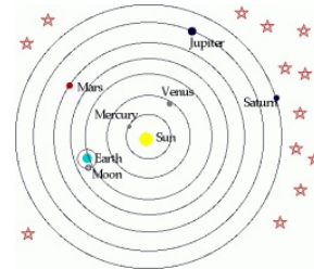
Heliocentrisk
