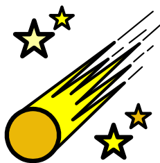
Komet
