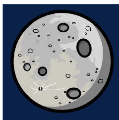
Månen
