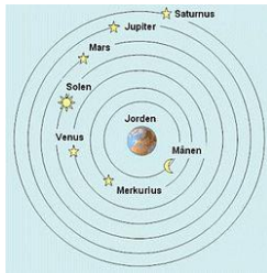
Geocentrisk
