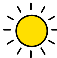
Solen
